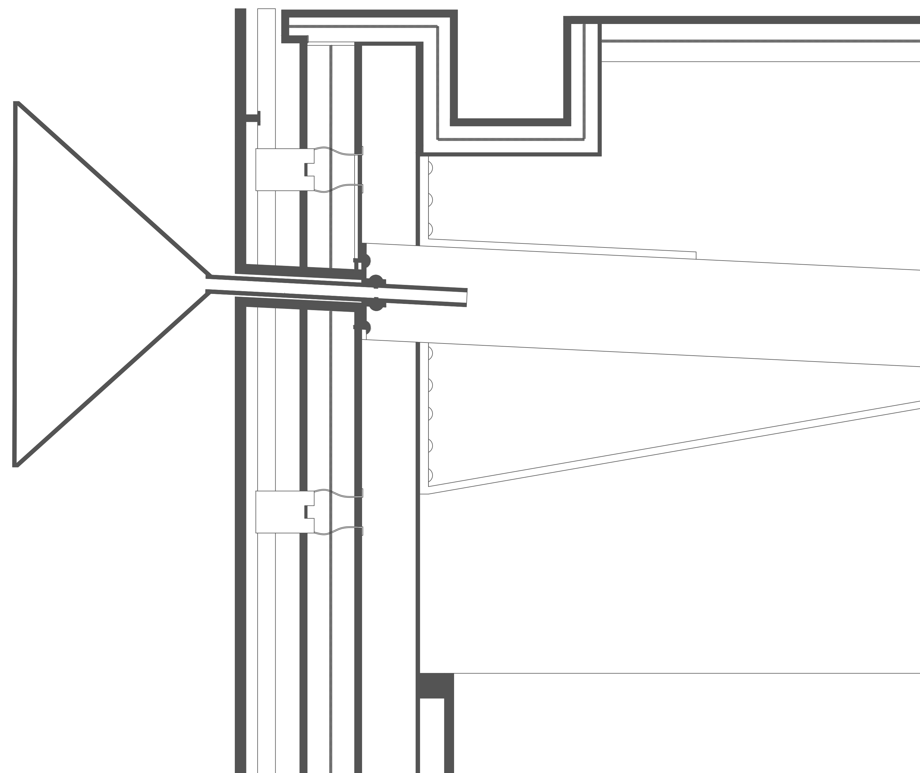
DÉTAIL FAÇADE AVEC SYSTÈME DE STOMATE OUVERTE
