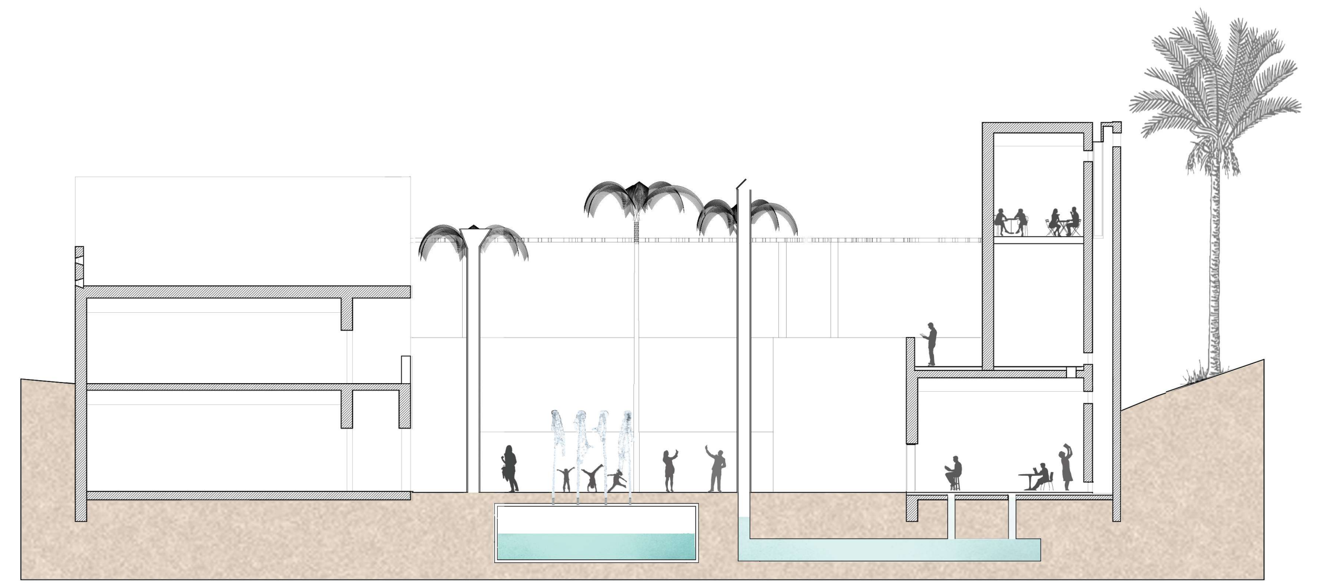
Coupe CC 1/200
