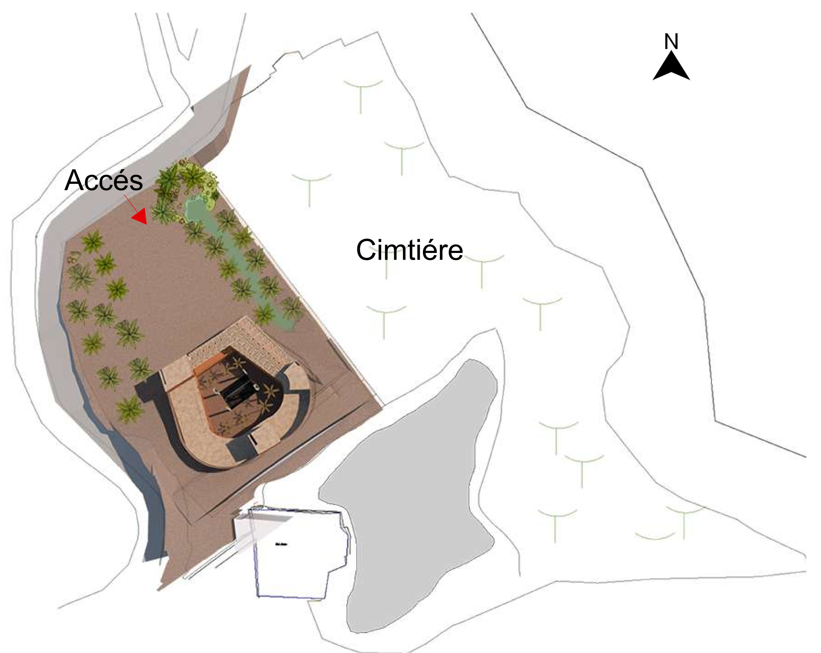
Plan de masse 1/1000
