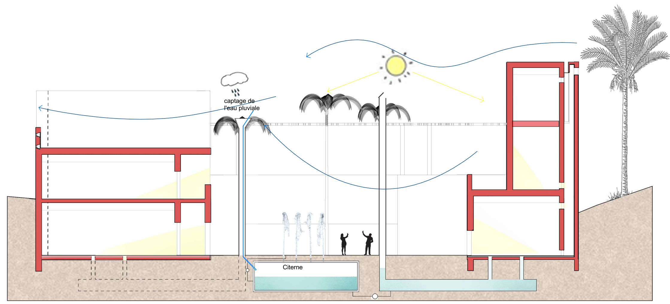
Coupe des principes bioclimatiques - Scénario hiver 1/200
