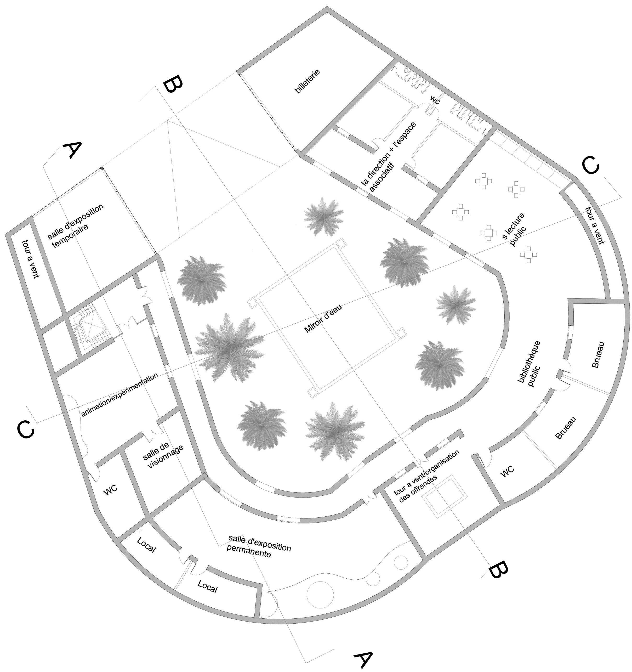
Plan RDC 1/200
