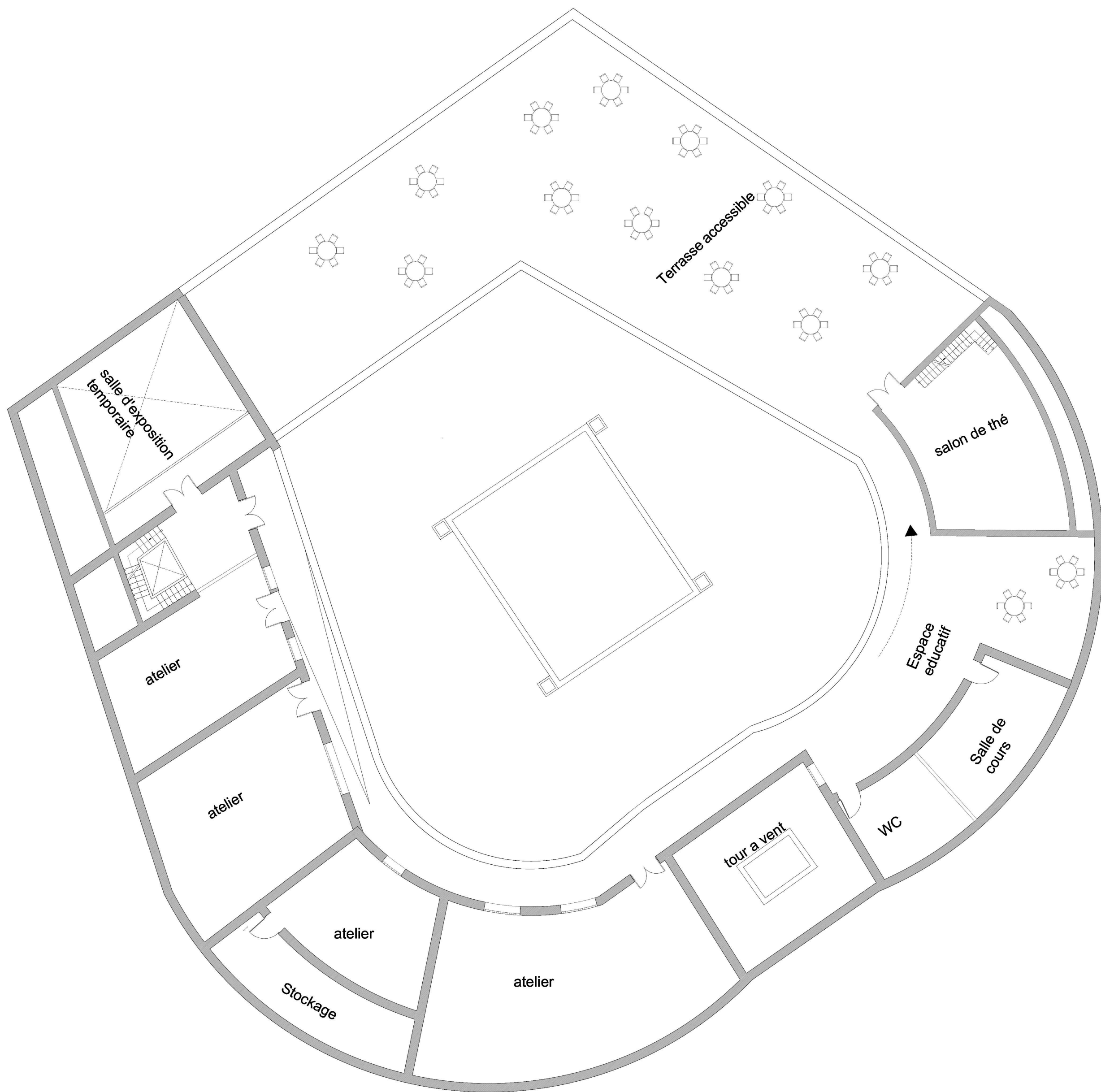
Plan RDC 1/200
