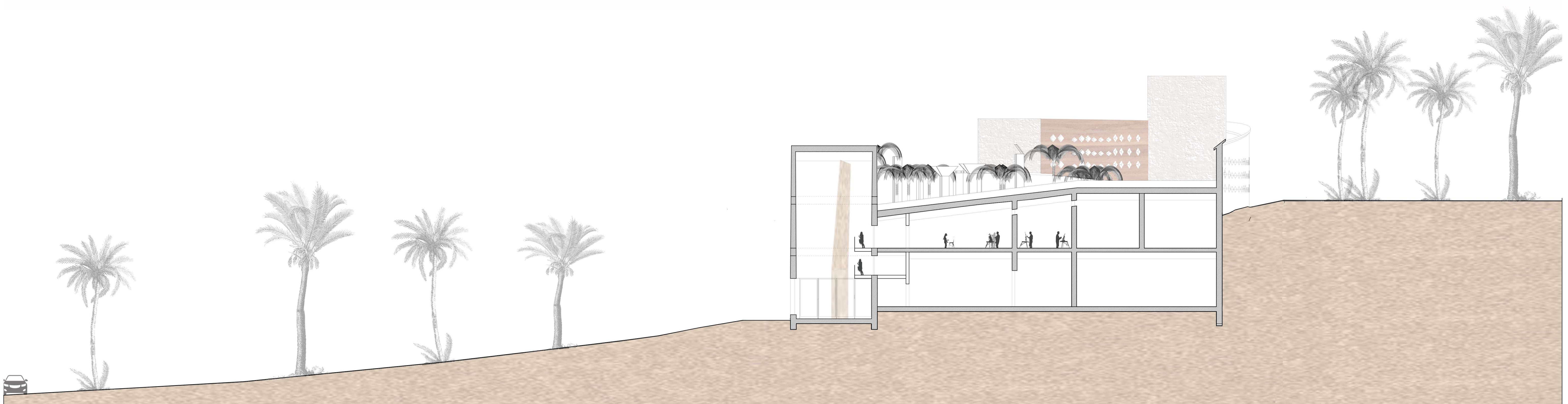
Coupe AA 1/200
